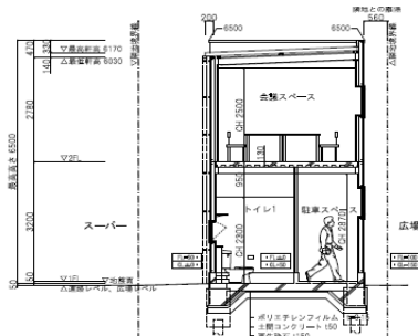
断面図 (短手)
