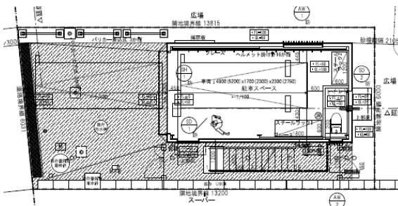
1階平面図
