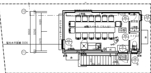
2階平面図
