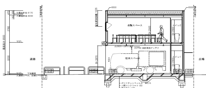
断面図 (長手)
